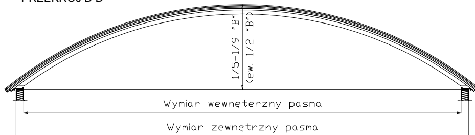
PASMO WIETLNE łUKOWE PRZEKRÓJ B-B
