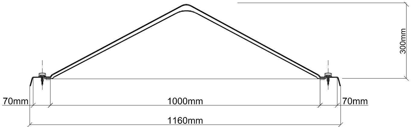
Kopułka podwójna
