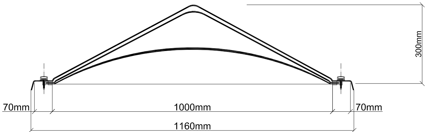
Kopułka potrójna
