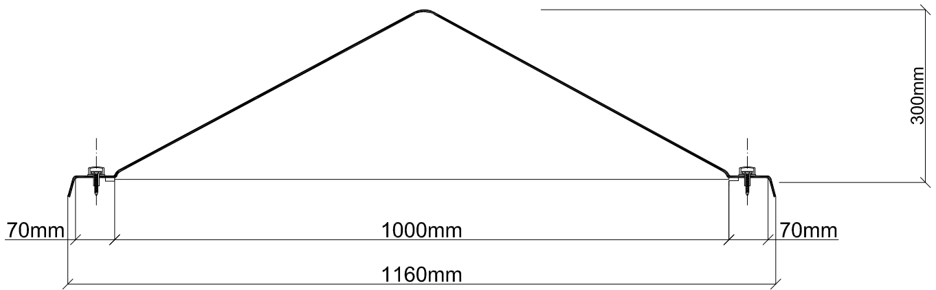
Kopułka pojedyncza
