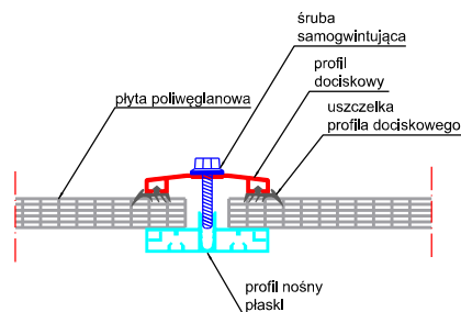
Połączenie płyt poliwęglanowych pokrycia pasma świetlnego
