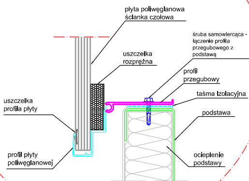
Mocowanie ścianki czołowej pasma świetlnego do podstawy
