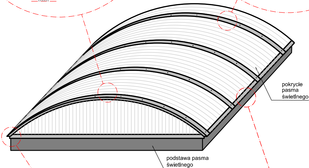
Mocowanie ścianki czołowej pasma świetlnego do podstawy
