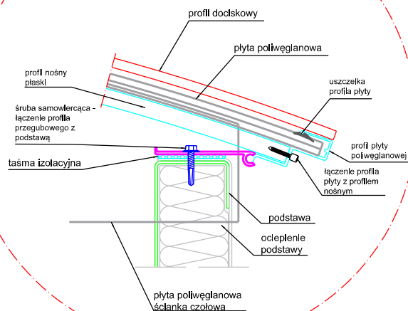
Mocowanie ścian bocznych pasma świetlnego do podstawy
