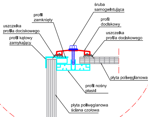
Mocowanie ściany czołowej z pokryciem pasma świetlnego
