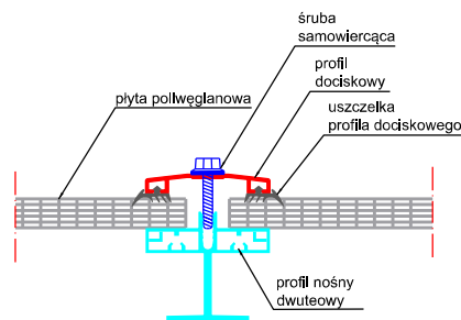
Połączenie płyt poliwęglanowych pokrycia pasma świetlnego
