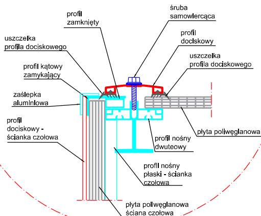
Mocowanie ściany czołowej z pokryciem pasma świetlnego
