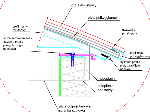
Mocowanie ścian bocznych pasma świetlnego do podstawy
