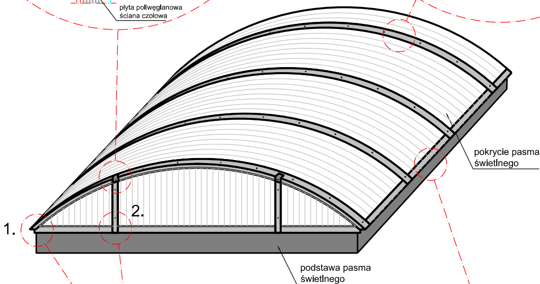
Mocowanie ścianki czołowej pasma świetlnego do podstawy
