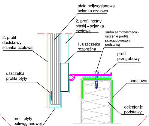
Mocowanie ścianki czołowej pasma świetlnego do podstawy
